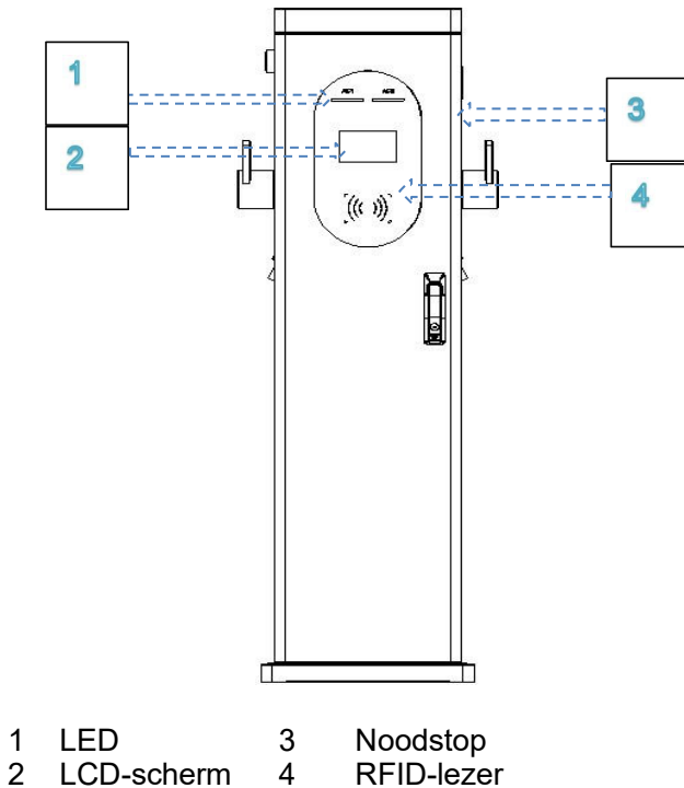
Fig. 4-1 HMI van AC EV-laadstation
